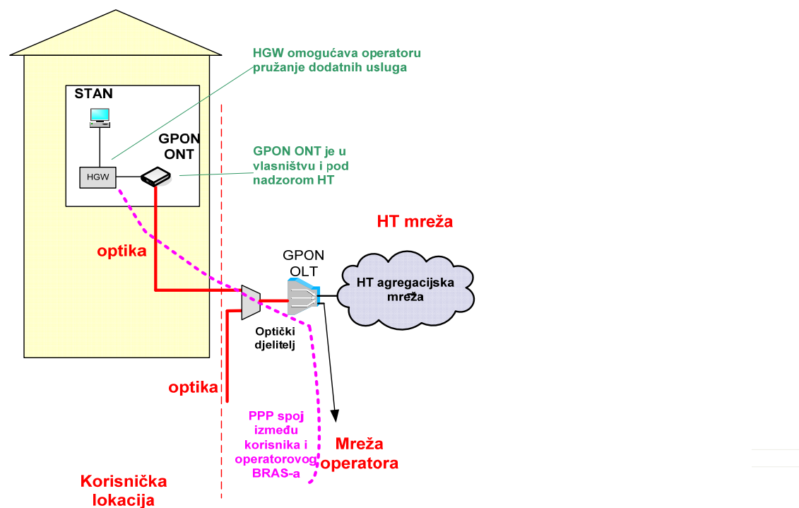
Slika 6. Način realizacije usluge veleprodajnog širokopojasnog pristupa za Internet uslugu na temelju FTTH rješenja na OLT razini
