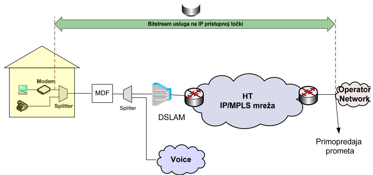
Slika 16. Veleprodajni širokopolasni pristup za pružanje VoIP usluge na IP razini u slučaju kada krajnji korisnik ostvaruje Osnovni pristup mreži putem usluge HT-a
